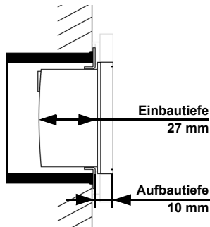
Abb. 2: Schnittzeichnung.
