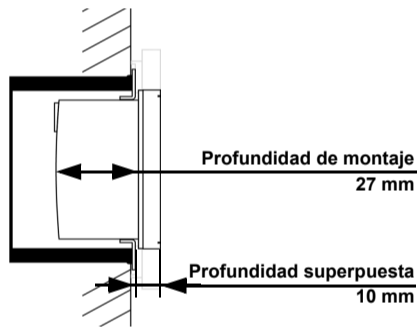
Fig. 2: Dibujo de sección. El Pulsador Cala KNX MultiTouch T se ajusta a una caja de dispositivos estándar ( \varnothing 60 mm, profundidad 42 mm). ¡El marco no está incluido en el volumen de suministro!
