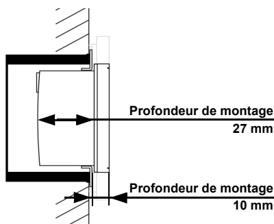
Fig. 1: Plan en coupe.
