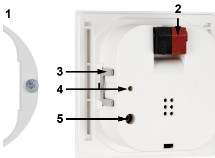
Abb. 2: Rückseite
