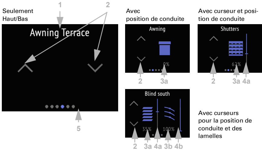
Fig. 16: Menu Moteur
