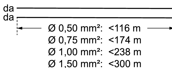
Figure 4: Longueur de ligne DALI
