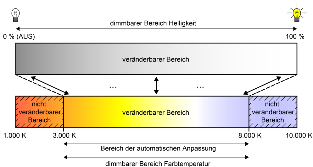
Bild 27: Automatische Anpassung der Farbtemperatur an die eingestellte Helligkeit Beispiel mit eingeschränktem Farbtemperaturbereich
