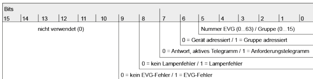
Bild 15: Telegrammaufbau 2-Byte-Fehlerstatus
