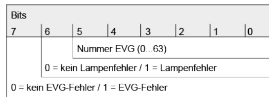
Bild 14: Telegrammaufbau 1-Byte-Fehlerstatus
