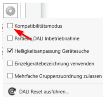
Bild 82: Kompatibilitätsmodus im Kontextmenü der DALI Inbetriebnahme
