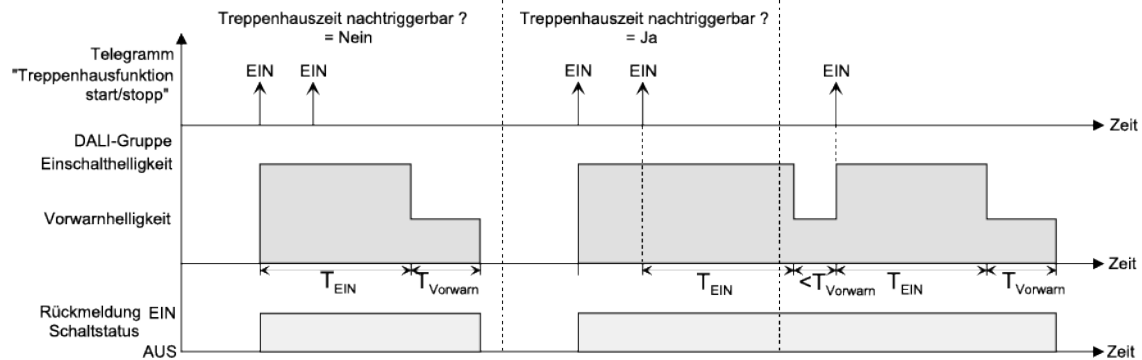
Bild 50: Einschaltverhalten der Treppenhaufunktion ohne Soft-Funktionen
