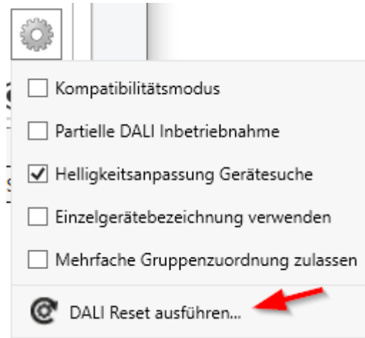
Bild 83: DALI Reset-Kommando im Kontextmenü der DALI Inbetriebnahme
