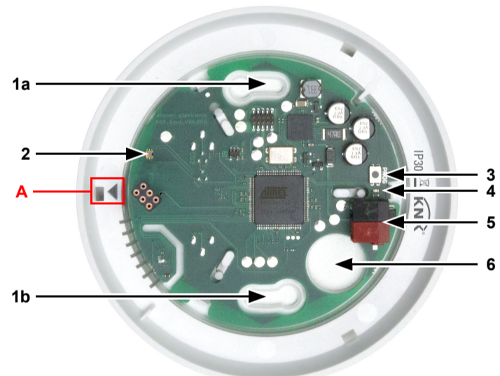
Fig. 1 1 a+b Asole per il fissaggio (Distanza foro 60 mm)
