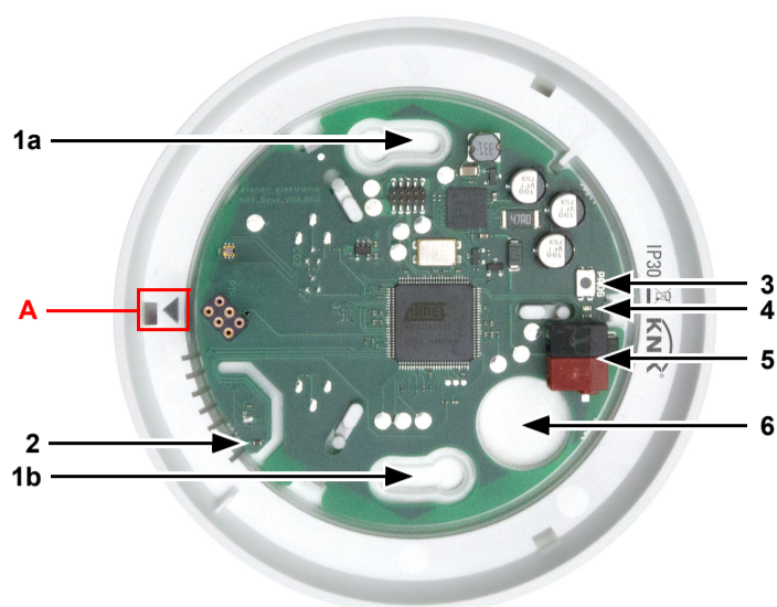
Fig. 1 1 a+b Asole per il fissaggio (Distanza foro 60 mm) 2 Sensore per temperatura 3 Tasto programmazione 4 LED programmazione 5 Morsetto KNX BUS +/- 6 Passaggio cavi A Marcatura per allineamento del coperchio
