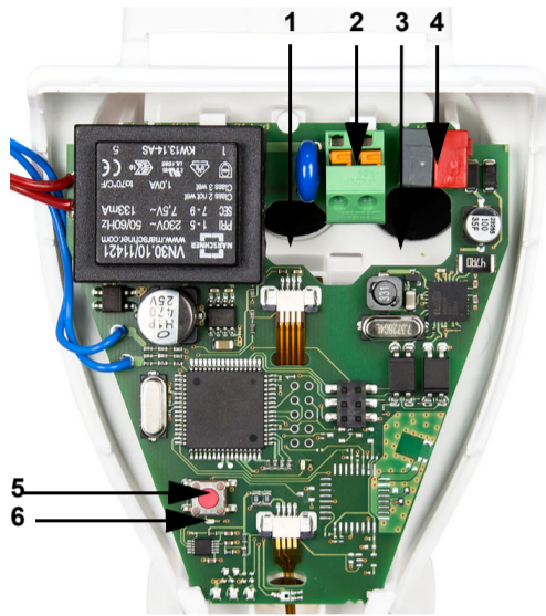
Fig. 11 1 Apertura para el cable de la fuente de alimentación 2 Clema de conexión rápida para la fuente de alimentación (230 V AC), apropiada para cable rígido de hasta 1,5 mm 2 o flexible. 3 Apertura para el cable de Bus 4 Clema de Bus KNX +/- 5 Botón de programación 6 LED de programación
