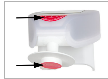
Fig. 16 Después de la instalación, retire la etiqueta protectora del sensor de viento y la etiqueta de información de "Distancia" en la parte superior de la cubierta.
