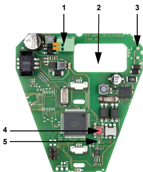
Fig. 12 1 Clema de conexión rápida para la fuente de alimentación (20...30 V DC), Cable rígido de hasta 1,5 mm 2 o flexible. Ocupación de bornes independiente de la polaridad (+/- o -/+) 2 Apertura para el cable de la fuente de alimentación, el cable de Bus 3 Conexión por clema de Bus KNX +/- 4 Botón de programación 5 LED de programación
