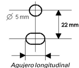
Fig. 8 a+b Esquema de taladrado
