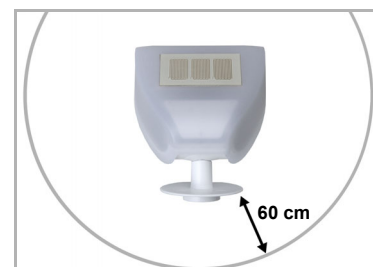
Fig. 1 La stazione meteo deve disporre di uno spazio libero sottostante, adiacente e frontale di almeno 60 cm (elementi o parti costruttive, ecc.).
