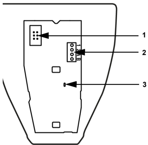
Fig. 12: Vista general de la placa de circuitos 1 Cable al sensor de lluvia en la cubierta del gabinete 2 Borne para la conexión 1: +24 V DC | 2: "-" A: Datos | B: Datos 3 LED de control por receptor GPS
