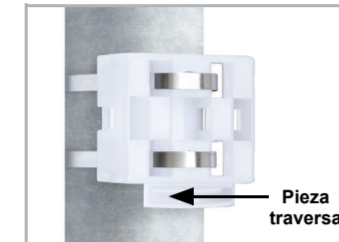
Fig. 6 Montaje en mástil: lado curvo hacia el mástil, la pieza travesera hacia abajo.
