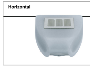
Fig. 3 La estación meteorológica se debe montar horizontalmente en la posición transversal.
