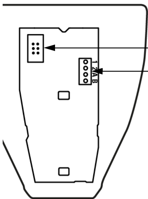
Fig. 12: Vista general de la placa de circuitos 1 Cable al sensor de lluvia en la cubierta del gabinete 2 Borne para la conexión 1: +24 V CC | 2: „-“ A: Datos | B: Datos
