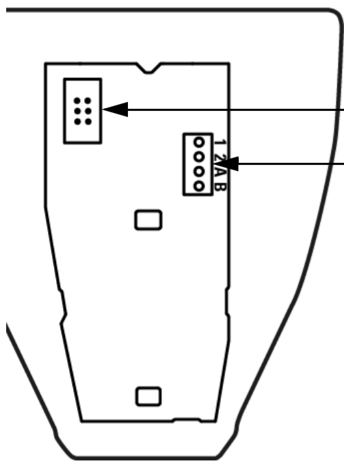
Abb. 12: Übersicht Platine
