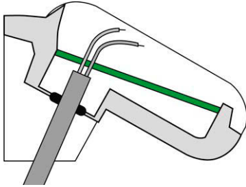
Abb. 17 Setzen Sie den Mantel des Kabels unterhalb der Platine ab und führen Sie nur die Anschlusskabel durch die Öffnungen in der Platine nach oben.
