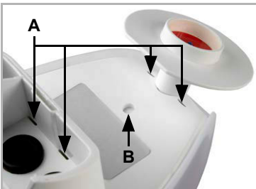
Abb. 22 (A) Auf der Gehäuseunterseite befinden sich Entwässerungsöffnungen. (B) Bei Bedarf, kann die zusätzliche, vorbereitete Entwässerungsstelle durchstochen werden. Gehen Sie dabei vorsichtig vor, um die innenliegende Platine nicht zu beschädigen.
