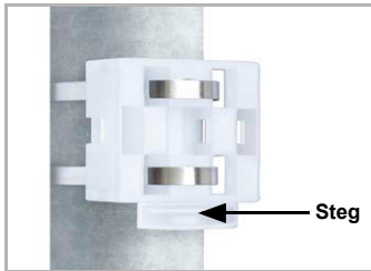
Abb. 11 Bei Mastmontage: geschwungene Seite zum Mast, Steg nach unten.
