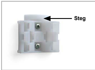
Abb. 10 Bei Wandmontage: ebene Seite zur Wand, halbmondförmiger Steg nach oben.
