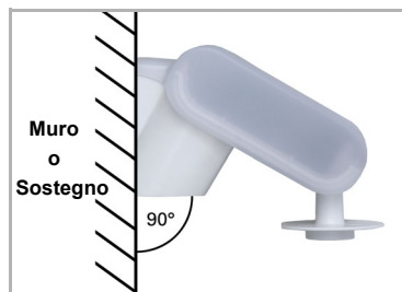
Fig. 2 Il sensore di vento deve essere applicato su un muro (o sostegno) verticale.
