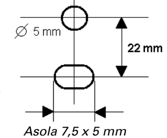
Fig. 8 a+b Disposizione fori.
