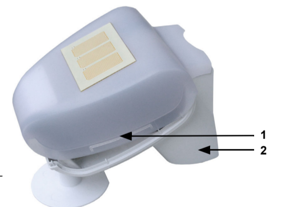
Fig. 9 1 Crans du couvercle 2 Partie inférieure du boîtier
