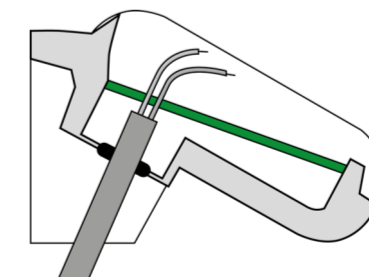
Fig. 10 Dénudez le câble au-dessous de la platine et introduisez uniquement les câbles de raccordement à travers les orifices dans la platine vers le haut.
