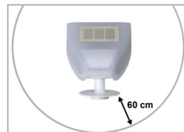
Fig. 1 Le détecteur doit avoir au-dessous, latéralement et sur le devant au moins 60 cm de distance avec les autres éléments (constructions, éléments de constructions, etc.).
