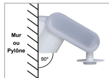
Fig. 2 Le détecteur de vent doit être installé sur un mur vertical (et/ou un pylône).
