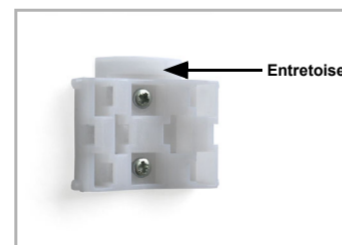
Fig. 4 Pour le montage mural : fixer le côté plan sur le mur, l'entretoise en forme de demi-lune doit être dirigée vers le haut.
